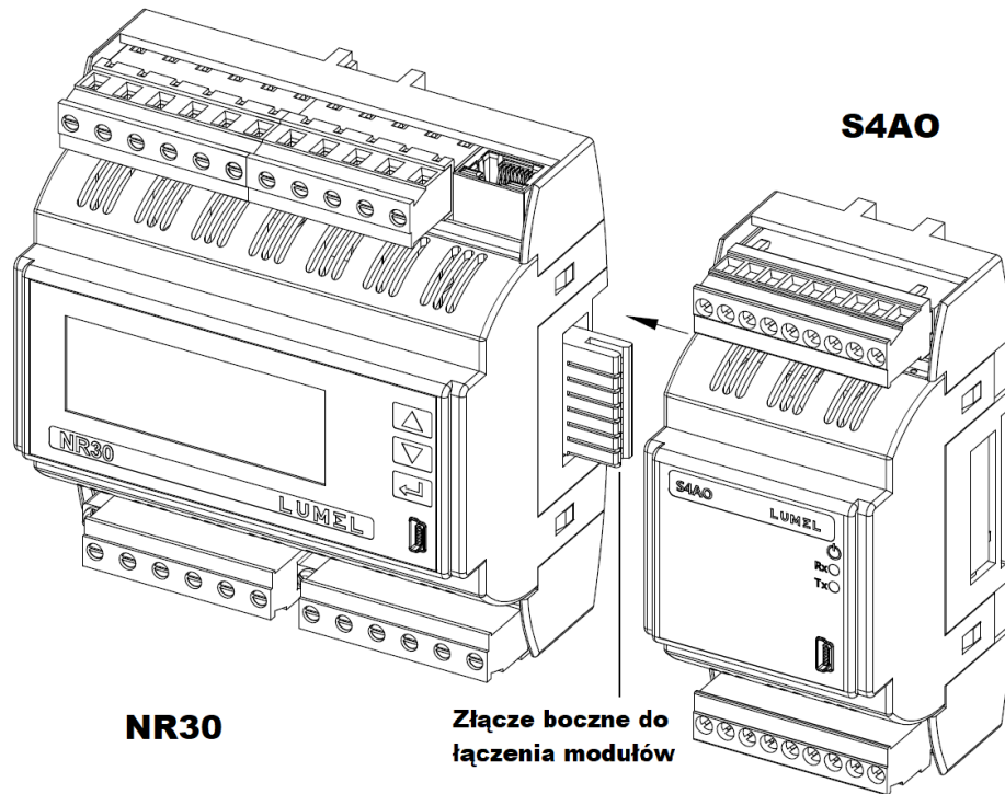
Rys.7. Łączenie modułów za pomocą złącza bocznego
