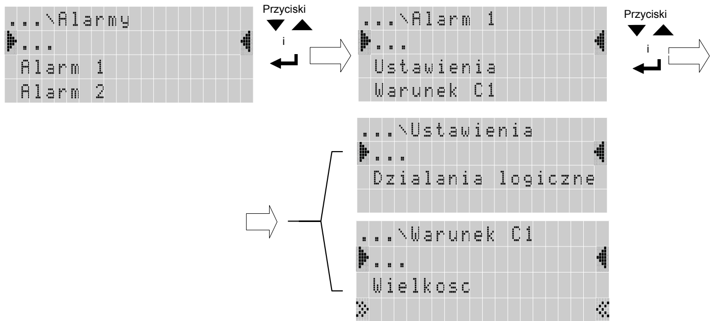
Rys.16. Ekran trybu Alarmy
