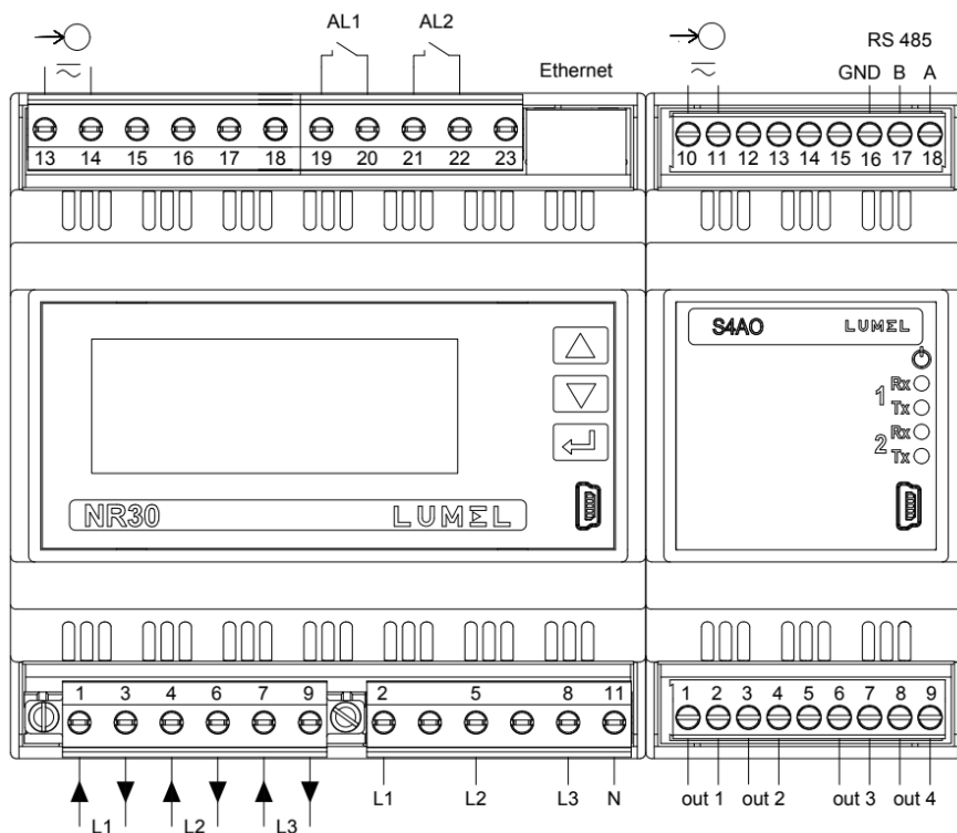
Rys.8. Podłączenie NR30 z S4AO interfejsem RS485
