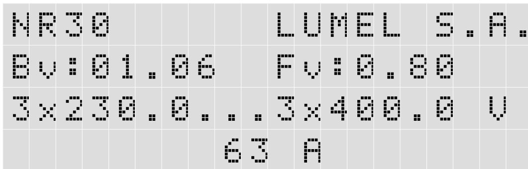
Rys.11. Ekran powitalny
